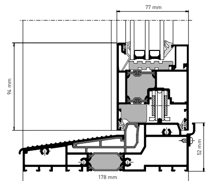
heroal S 77 HI (HS-Flügelprofil 77/94)
