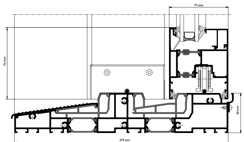
heroyal S 77 Schnittdarstellung Bodenschwelle dreispurig [HS-Flügelprofil 77/94]
