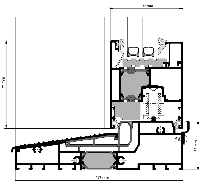
heroal S 77 HI Schnittdarstellung Bodenschwelle zweispurig (HS-Flügelprofil 77/94)
